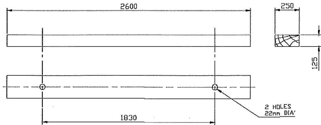
TYPE 1 Item 30093
